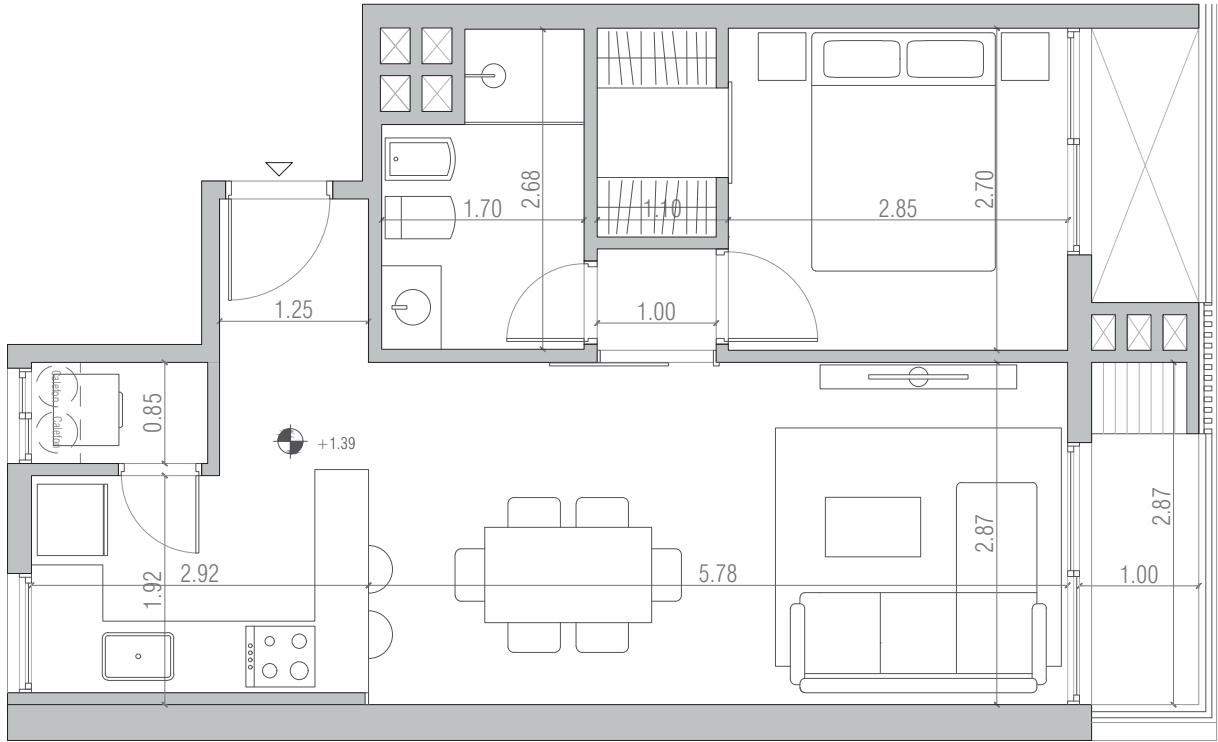
UNIDAD 101 - 1D APPCU 59m 2
