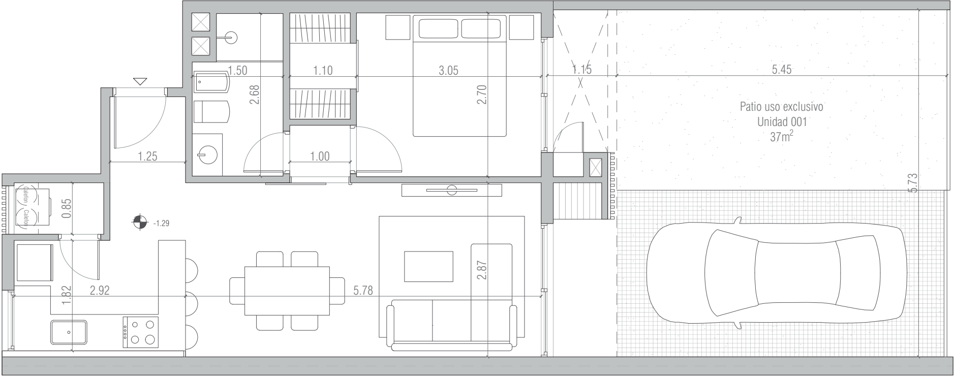
UNIDAD 001 - 1D APPCU 112m 2
