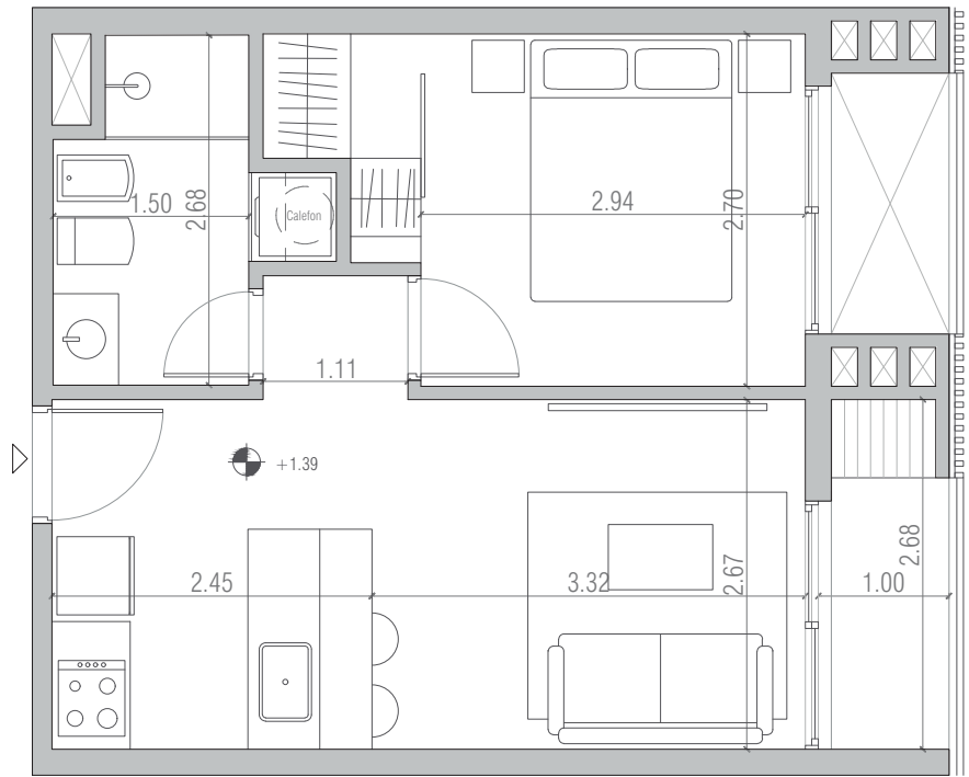
UNIDAD 102 -1D APPCU 46m 2
